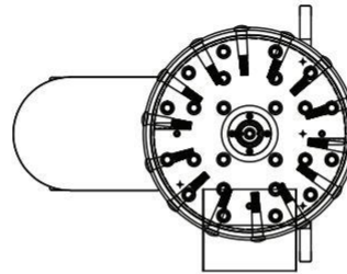
CP 1500 GB- Footprint
