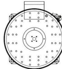
CP 1500 GB- Footprint
